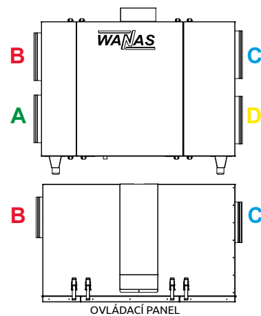
OVLÁDACÍ PANEL LEVÁ VERZE
